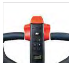
Pulsante bassa velocità Indicatore LED per batteria scarica Sbloccaggio del carrello elevatore con codice PIN a quattro cifre
